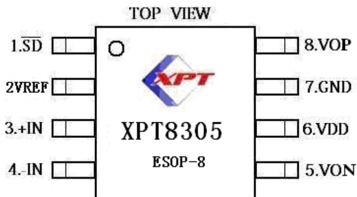
XPT8305 ESOP8 封装的管脚分布图
