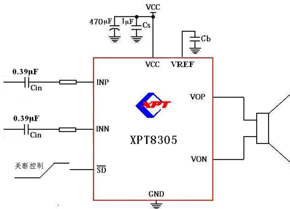
差分输入应用电路
