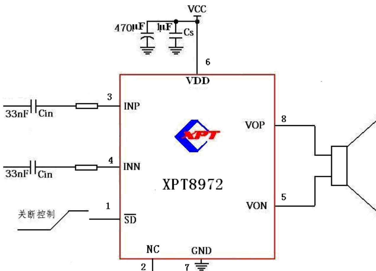
图1 差分输入应用电路
