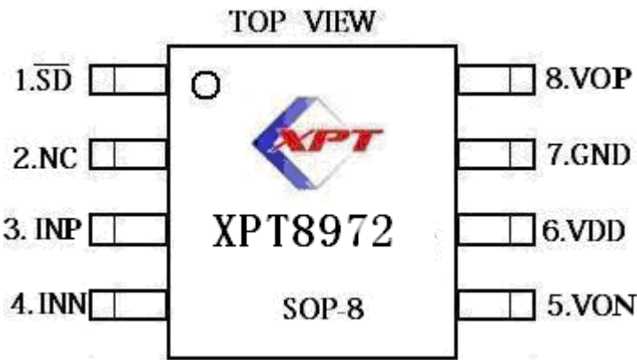
图 2 XPT8972 SOP8 封装的管脚分布图
