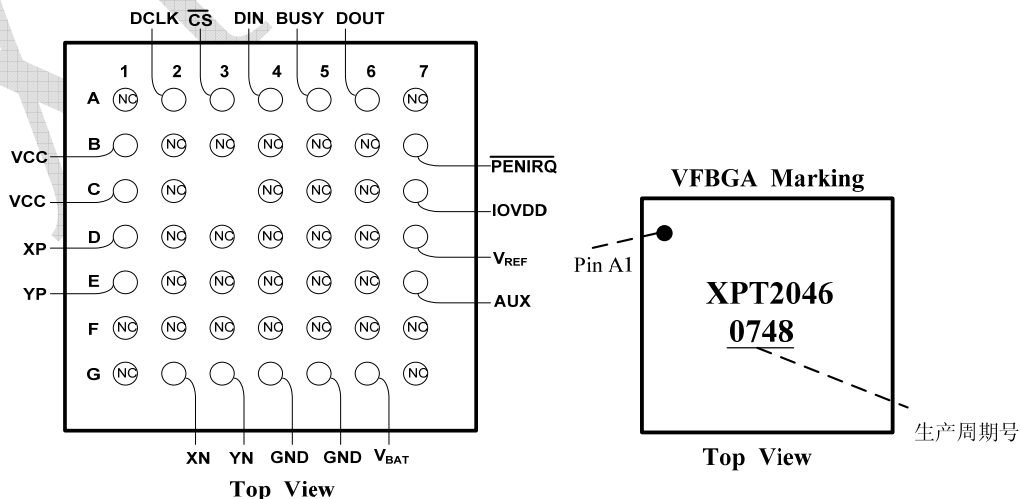
图4 XPT2046 的 VFBGA-16 封装管脚 (产品代号: XPT2046IZQCR)
