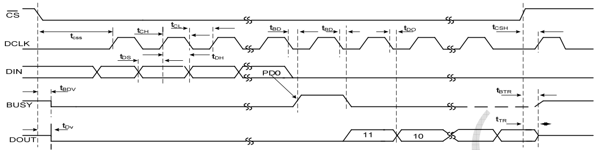
图15 详细时序图
