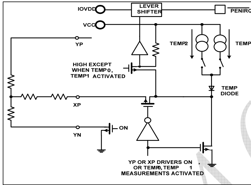
图13 PENIRQ 功能模块图
