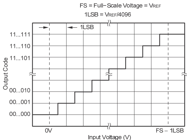
图17 理想情况输入电压和输出编码对应关系
