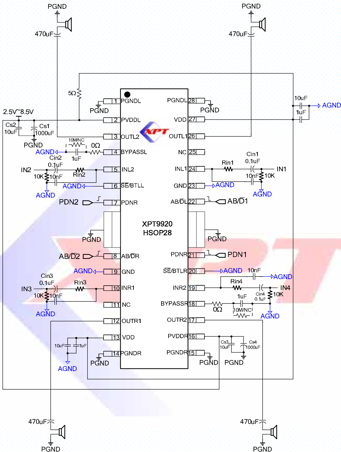
XPT9920 四声道典型应用图
