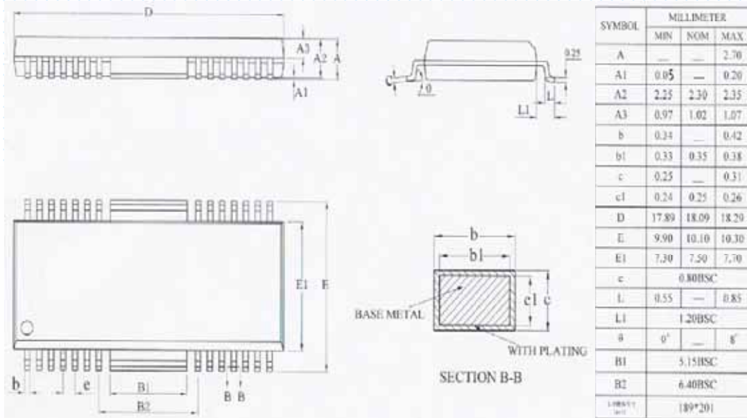
HSOP28 封装尺寸图
