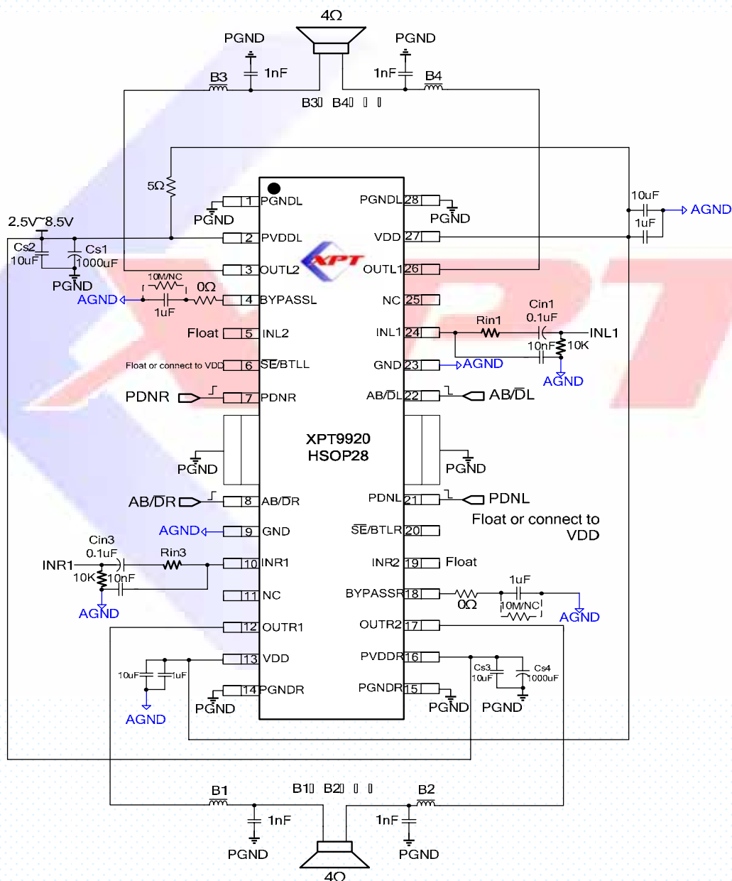
XPT9920 双声道典型应用图
